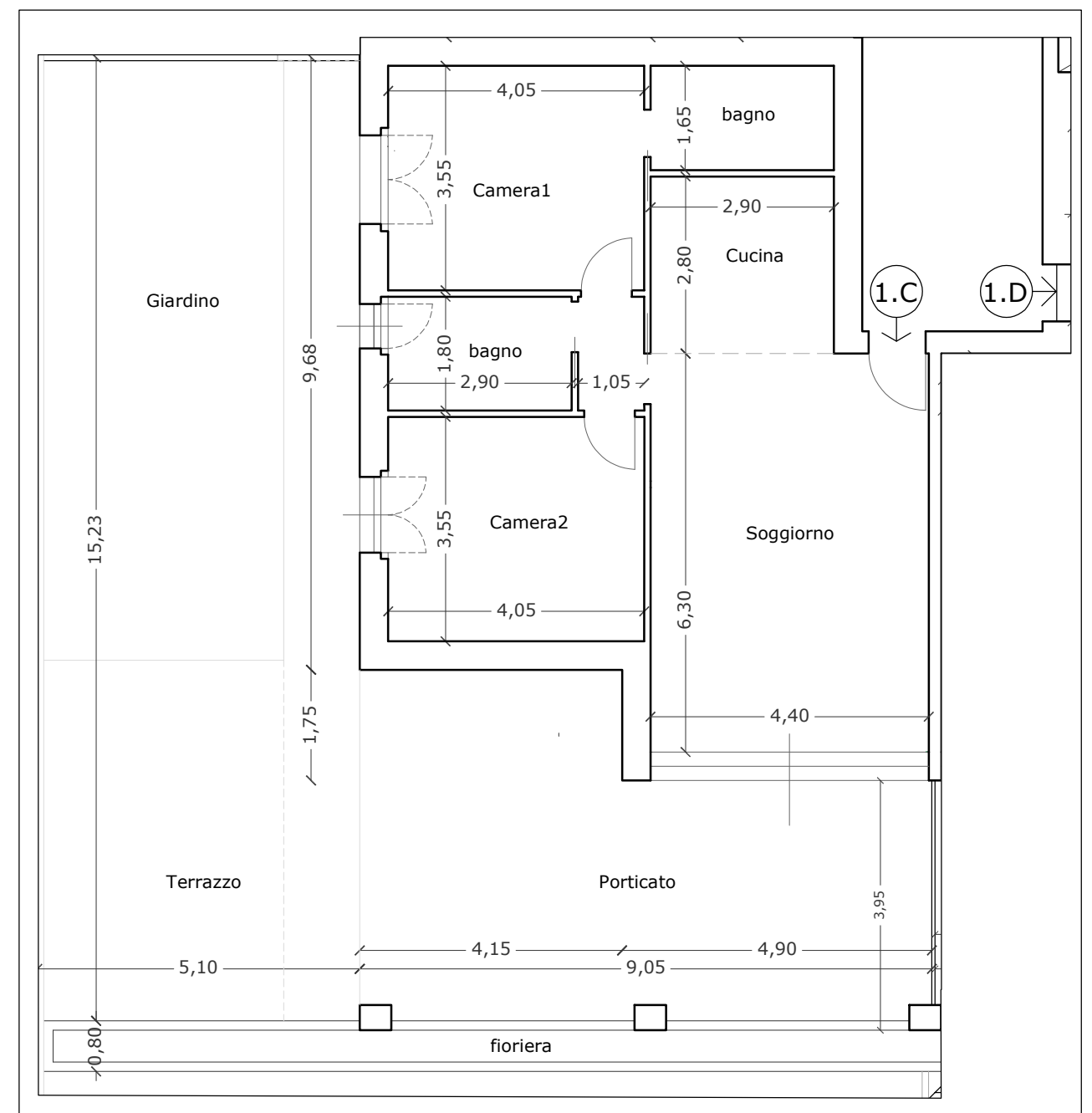
PIANO TERRA / RIALZATO
